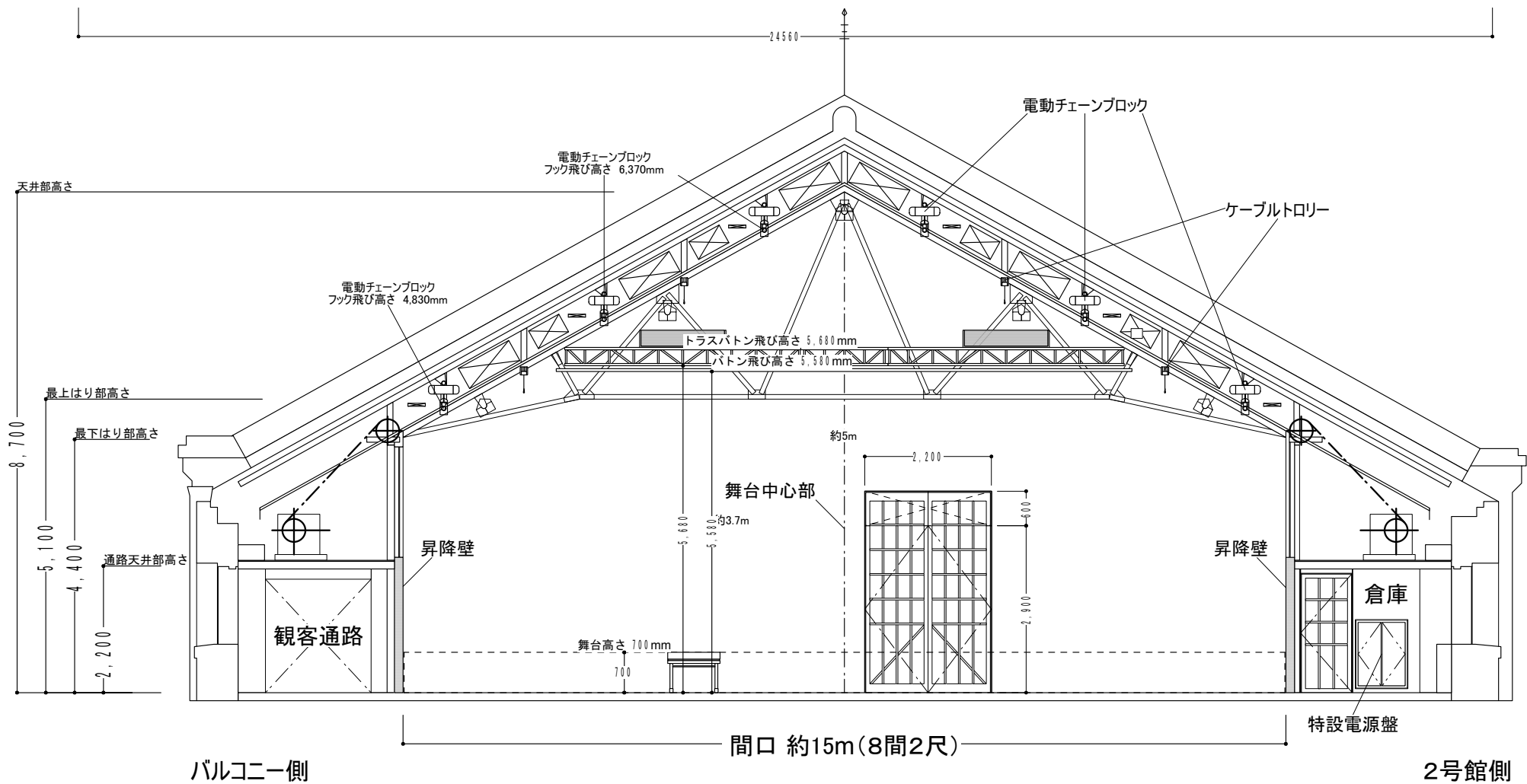
3階ホール 舞台断面図 1/100 (A3)
